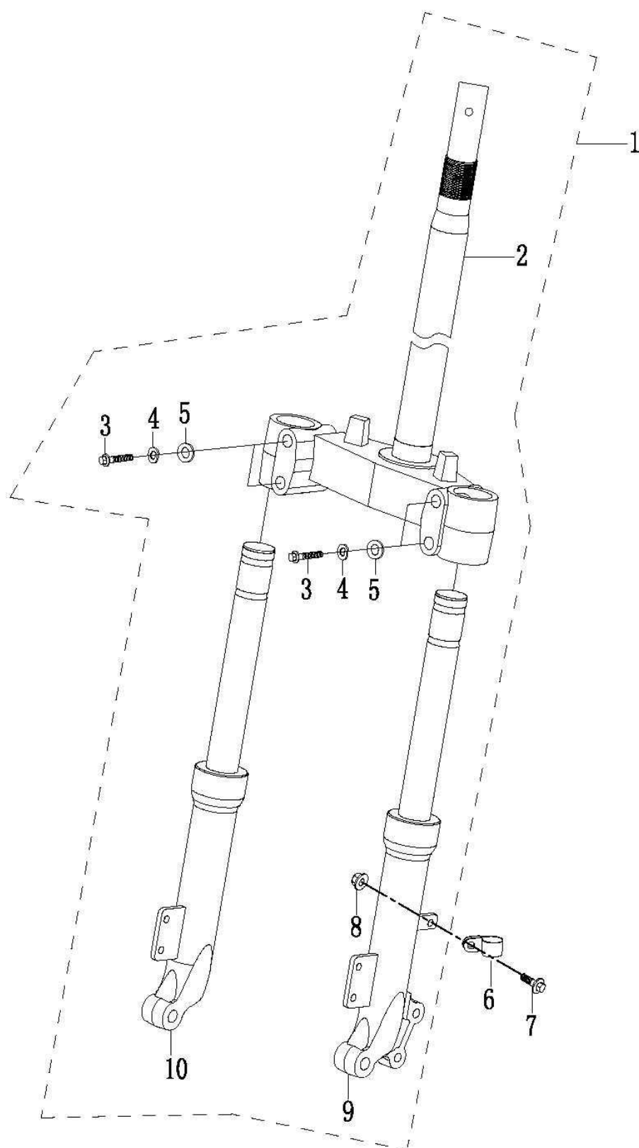
6-Steering/front shock
